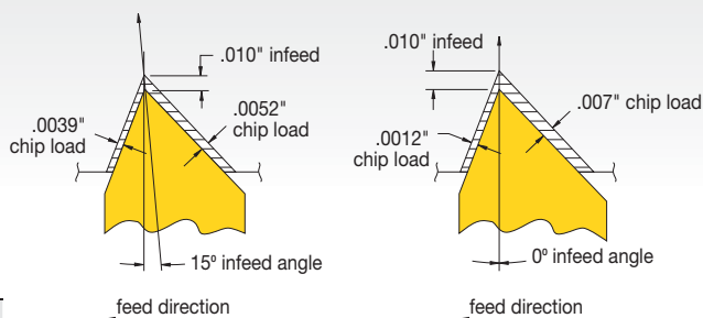
NTB-A insert
