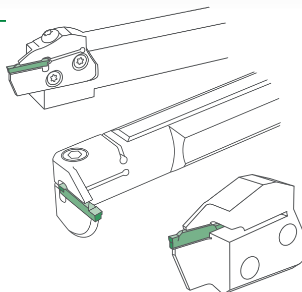
FACE GROOVING
